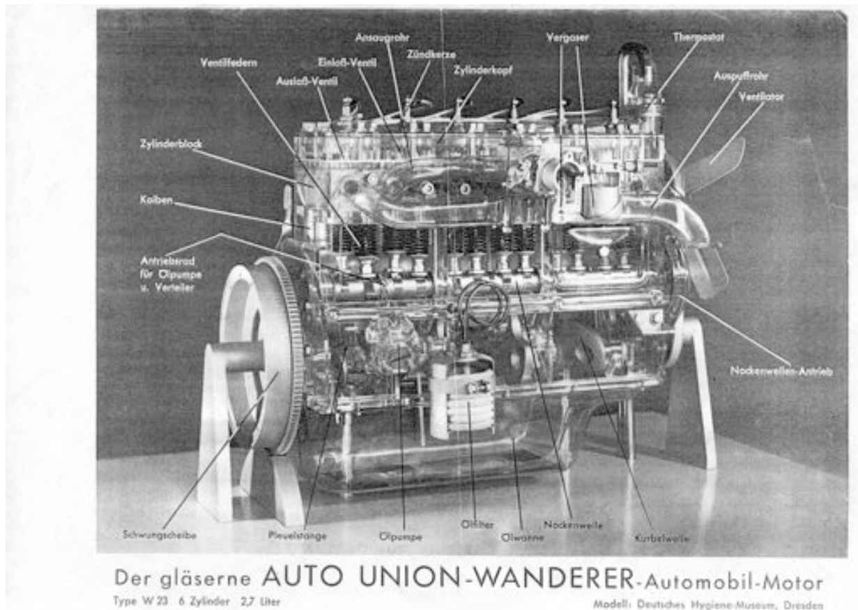
Abb. 12 Das Modell zeigt den Motor des von 1937-1940 hergestellten Auto Union Wanderer W23 (Abb.: Archiv des Deutschen Hygiene Museums).
